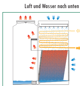
Mehrstromprinzip
