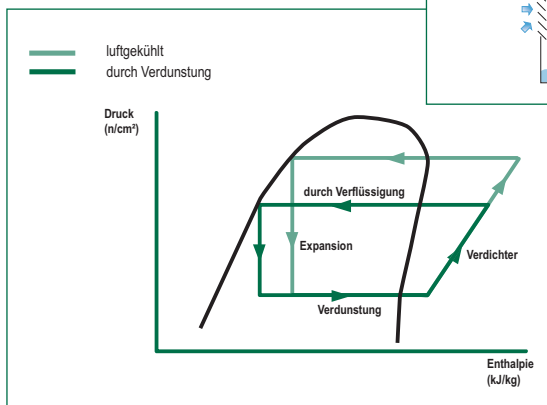
Mehrstromprinzip
