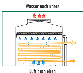
Gegenstromprinzip
