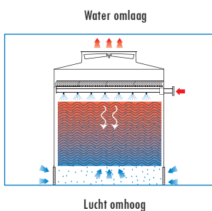
Tegenstroom
