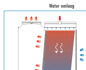
Kruisstroom
