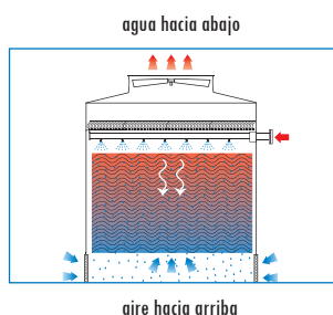
Configuración flujo a contracorriente
