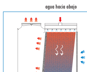
Configuración flujo cruzado
