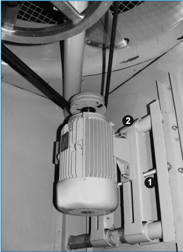
Chaise de moteur réglable
