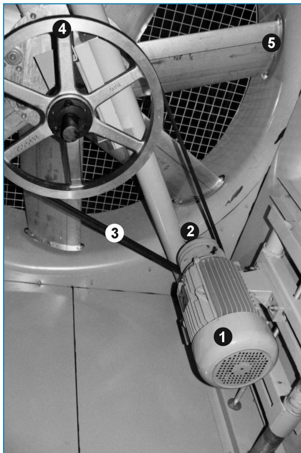
Aandrijfsysteem
